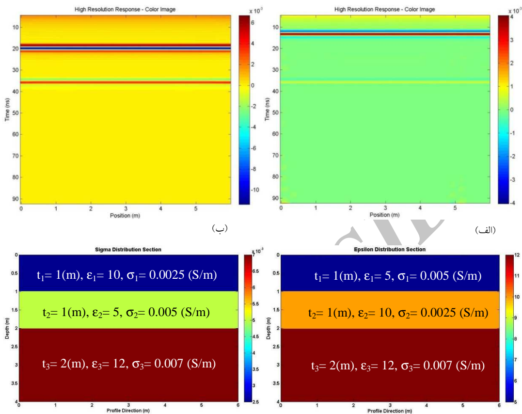
شکل ۴. تاثیر تغییرات توام گذردهی دی الکتریک و هدایت الکتریکی بر پاسخ GPR. برای دو مدل زمین سه لایه‌ای. مدل الف - \epsilon_2 = 2\epsilon_1, \sigma_2 = 0.5\sigma_1 ؛ مدل ب - \epsilon_2 = 0.5\epsilon_1, \sigma_2 = 2\sigma_1 (هدایت الکتریکی برحسب زمینس بر متر می باشد).
