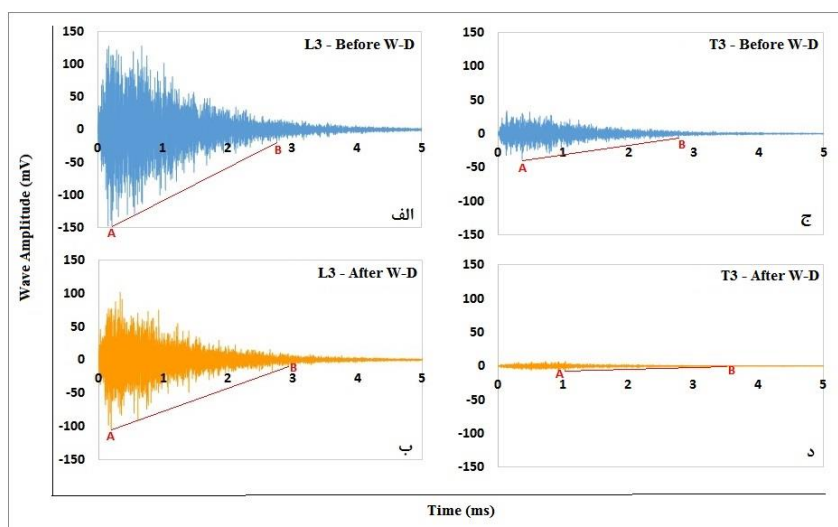
شکل ۸. نمودار امواج التراسونیک دریافتی از نمونه‌های L3 و T3 قبل و بعد از چرخه‌های تر و خشک شدن
