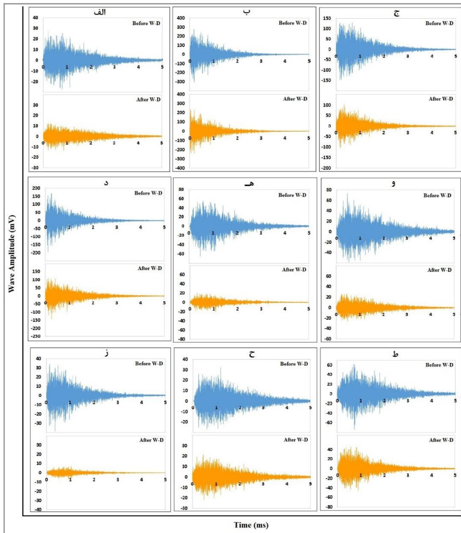
شکل ۶. نمودار امواج التراسونیک دریافتی از نمونه‌ها قبل و بعد از چرخه‌های تر و خشک شدن. الف L1، ب L2، ج L3، د L4، ه T1، و T2، ز T3، ح T4، ط T5
