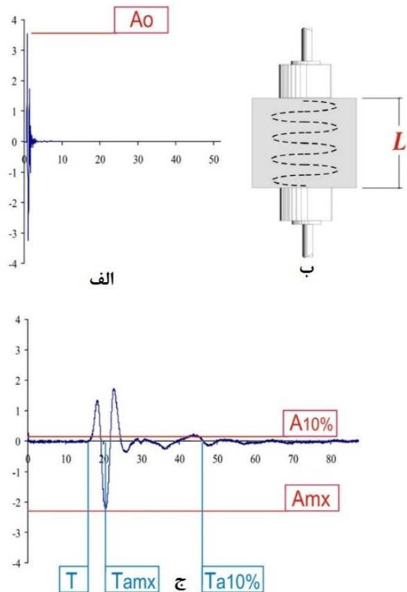
شکل ۳. الف) دامنه حداکثر موج ارسال شده به نمونه، ب) وضعیت قرارگیری نمونه و مبدل‌های فرستنده و گیرنده، ج) نمودار موج دریافت شده از نمونه و نحوه تعیین A_{10\%} ، A_{max} ، T_{10\%} و T_{max} از نمودار موج (Martínez-Martínez et al., 2011)
