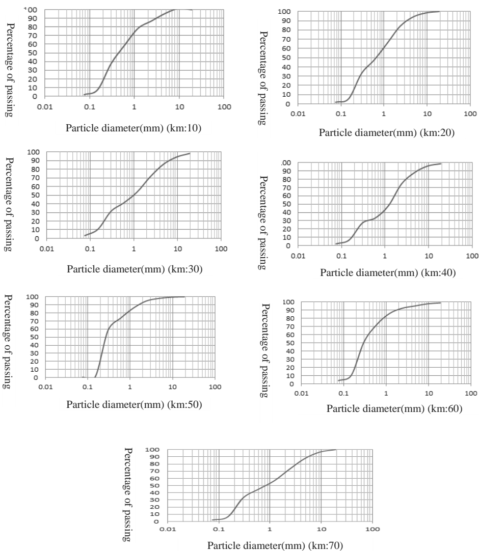
شکل ۴. منحنی‌های دانه بندی
