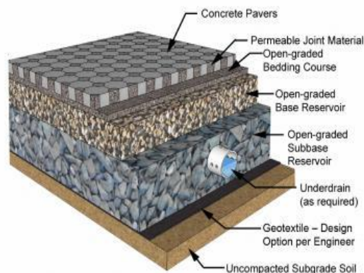
شکل ۳. نمایی از لایه های مختلف روسازی نفوذپذیر (کمالی و تجربی، ۱۳۹۰)
