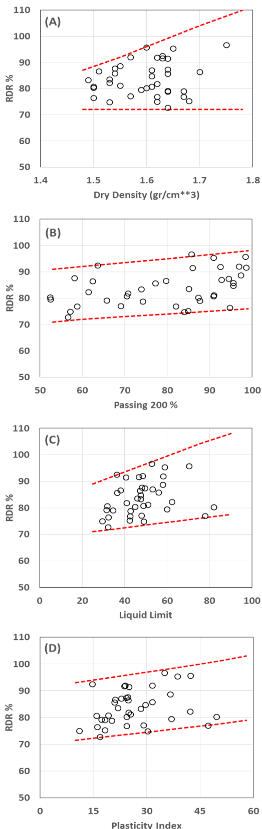
شکل ۷. نسبت کاهش مقاومت الکتریکی خاک به ازای رطوبت ۲۵ درصد در مقابل مشخصات فیزیکی خاک
