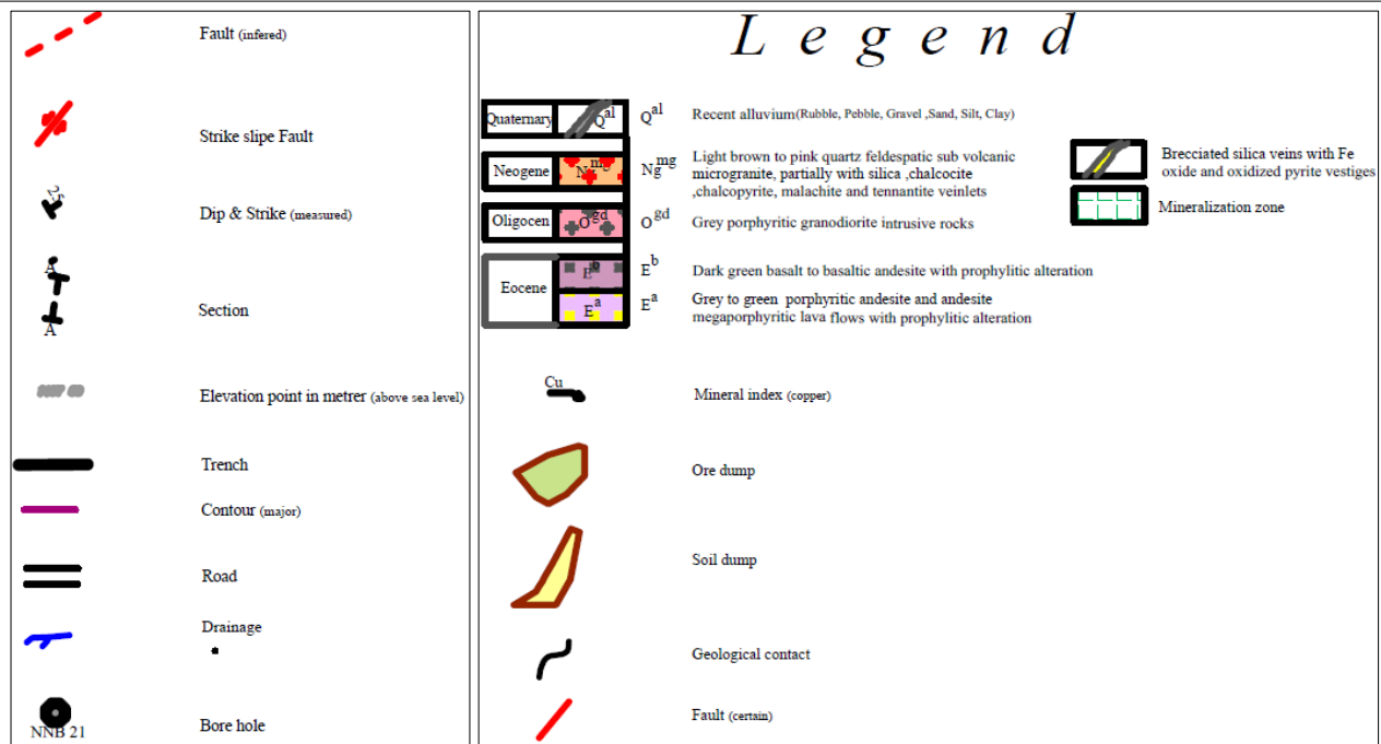
شکل ۱. نقشه زمین شناسی ۱:۱۰۰۰ محدوده کانسار نارباغی شمالی همراه با نمایش موقعیت گمانه ها و ترانسه های اکتشافی (برگرفته از پیچاب کانسار، ۱۳۹۴).
