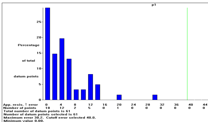
شکل ۸. خطای مجذور میانگین مربعات (RMS) در محاسبه مقاومت ویژه ظاهری بلوک‌های مختلف پروفیل P1.
