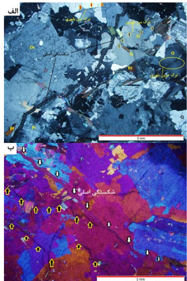
شکل ۹. تصاویر مقطع نازک تهیه شده در راستای عمود بر شکستگی اصلی الف: نمونه GD1 و ب: نمونه GD2
