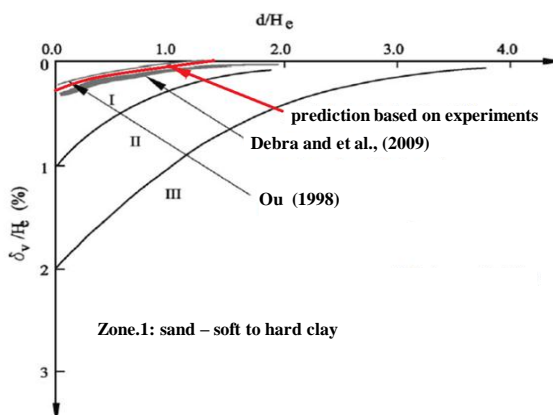
شکل ۱۳. نشست زمین مجاور گود
