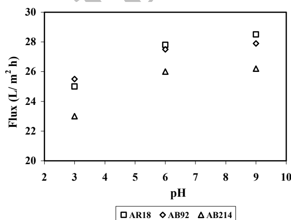
شکل ۹: تغییر شار عبوری در مقادیر مختلف pH برای رنگزاهای گروه سوم (غلظت رنگزا=۲۰۰ ppm، فشار=۴ بار، زمان=۳۰ دقیقه).
