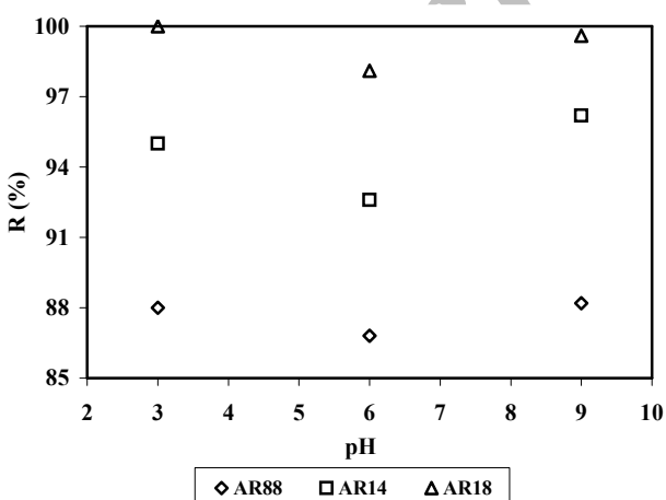
شکل ۱۲: تغییر احتباس در مقادیر مختلف pH برای رنگزاهای گروه چهارم (غلظت رنگزا=۲۰۰ ppm، فشار=۴ بار، زمان=۳۰ دقیقه).
