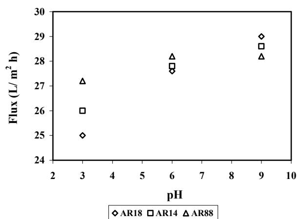
شکل ۱۱: تغییر شار عبوری در مقادیر مختلف pH برای رنگزاهای گروه چهارم (غلظت رنگزا=۲۰۰ ppm، فشار=۴ بار، زمان=۳۰ دقیقه).
