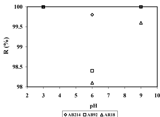
شکل ۱۰: اثر pH بر احتباس رنگزاهای گروه سوم (غلظت رنگزا = ۲۰۰ ppm، فشار=۴ بار، زمان=۳۰ دقیقه).
