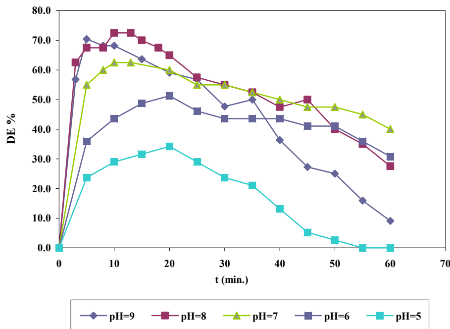
شکل ۴: درصد حذف رنگینه برای رنگینه سیاه راکتیو ۵ با غلظت ۴۰ ppm در HRT برابر با ۶۰ دقیقه، دمای محیط، فعالیت آنزیمی ۵ U/ml، غلظت آب اکسیژنه برابر با ۹۶.۱ mM و pH های متفاوت.
