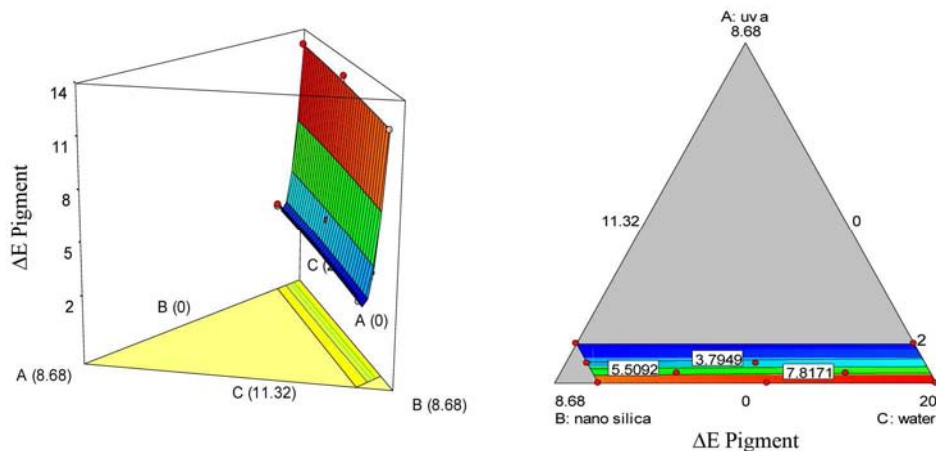
شکل ۷: نمودارهای سطح پاسخ و تاثیر فاکتورها بر ثبات نوری.
