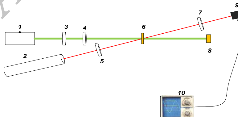
شکل ۴: چیدمان دو شکستی القاء لیزری: (۱) لیزر Nd:YAG 532 \text{ nm} (۲) لیزر هیلیوم-نئون 633 \text{ nm} (۳) قطبش‌گر 45^\circ (۴) روزنه، (۵) قطبش‌گر 45^\circ (۶) نمونه، (۷) قطبش‌گر 45^\circ (۸) جاذب، (۹) آشکارساز، (۱۰) اسیلوسکوپ.
