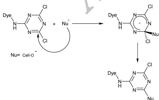
شکل ۱: واکنش جانشینی هسته دوستی در گروه واکنش‌پذیر دی کلرو تری آزین (X گروه هسته دوست).
