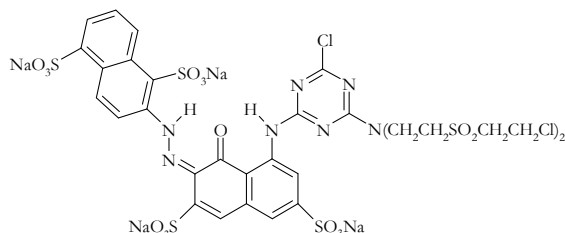
شکل ۱۸: رنگزاهای راکتیو سه عاملی رمازول رد اس بی بی.
