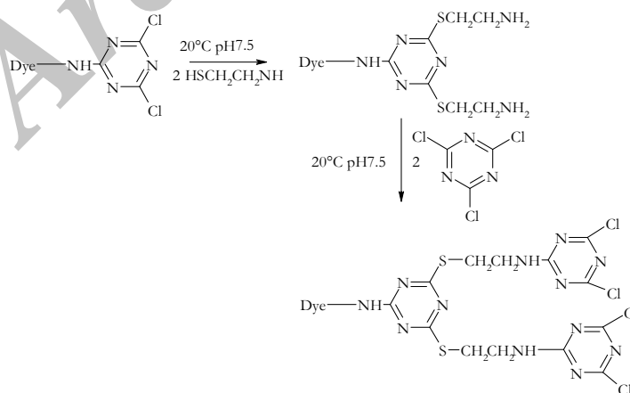
شکل ۲۰: روش سنتز برای رنگزاهای راکتیو چهار عاملی کلرو تری آزین دارای گروه اتصال‌دهنده سیستی آمین.
