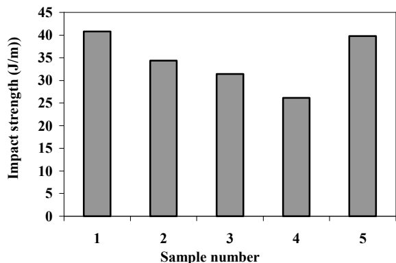
شکل ۶: نتایج استحکام ضربه برای نمونه‌های آمیزه چوب-پلاستیک.
