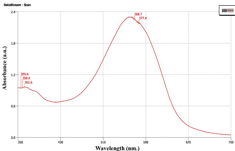
شکل ۳: طیف مرئی - فرابنفش ماده رنگزا در حلال DMSO.
