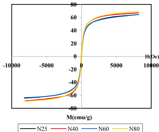
شکل ۳: منحنی هیستریز مغناطیسی در جو نیتروژن.
