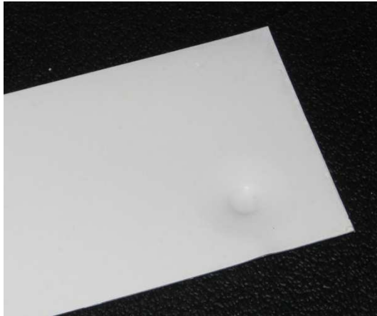
شکل ۸: تصویر از سطح نمونه D (رنگ با نسبت رنگدانه به رزین ۳:۱) پس از انجام آزمون ضربه.
