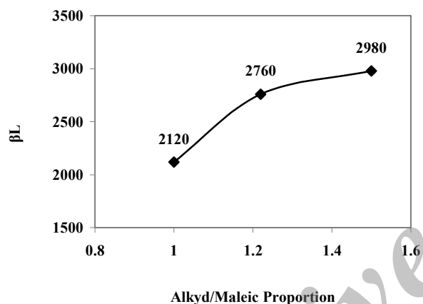
شکل ۱۱: منحنی شدت فلورسانس مخلوط رزین آلکید بلند روغن و ورنی مالئیک حاوی ۰,۵٪ رنگزای D.Y.۲۳۲ برحسب درصد اختلاط دو رزین. (روش محاسبه اختلاف سطح زیر دو منحنی انعکاسی می باشد).
