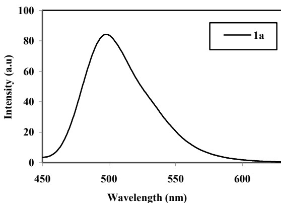
شکل ۱: طیف نشری رنگزای D.Y.232 در حلال استونیتریل (غلظت 10^{-5} mol Lit ^{-1} ) با فیلتر ۱٪ و تصویر محلول در همان حلال در نور روز (۱) و نور UV (۲).
