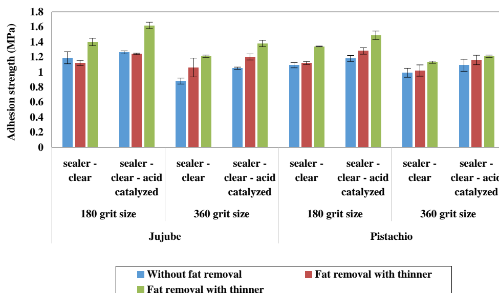
شکل ۳: مقایسه تأثیر متقابل نوع گونه چوبی، پرداخت سطح چوب، چربی زدایی سطح و نوع پوشش بر مقاومت چسبندگی.
