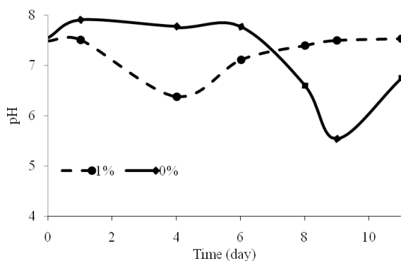
شکل ۸: تغییرات pH و کدورت محیط‌های کشت حاوی باکتری تیوباسیلوس تیوپاروس نسبت به زمان پس از ۳ دوره تابش و تاریکی در حضور نمونه‌های سیمانی عاری و حاوی ۱٪ نانوذرات دی‌اکسید تیتانیم.
