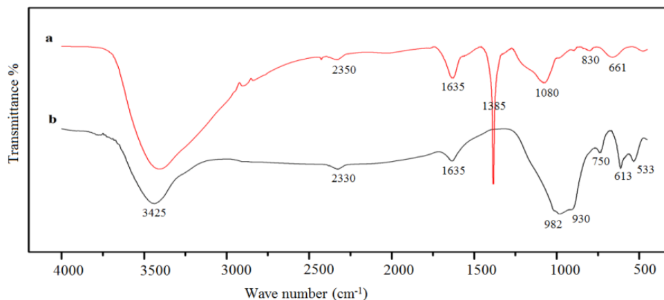
شکل ۲: طیف FTIR از نمونه GNNaF (a) در حالت ژل و (b) کلسینه شده در 1200\text{ }^\circ\text{C} .
