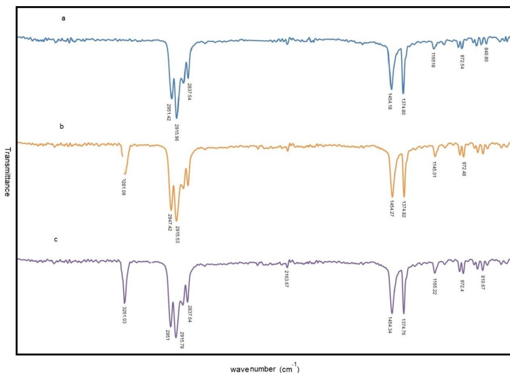
شکل ۴: مقایسه طیف FTIR-ATR (a) پلاسما نشده (b) پلاسما شده با اکسیژن (c) پلاسما شده با اکسیژن-آرگن.
