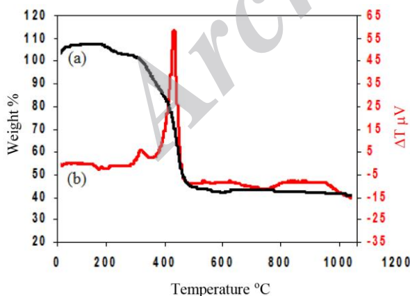
شکل ۳: (a) منحنی TGA و (b) منحنی DTA مربوط به پیش ماده کمپلکس معدنی.
