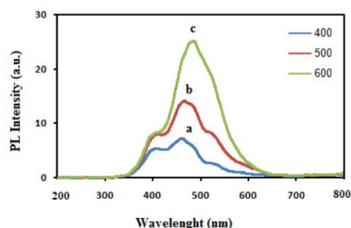
شکل ۷: طیف PL نانوذرات سنتز شده در دماهای مختلف (a) ۴۰۰°C، (b) ۵۰۰°C و (c) ۶۰۰°C.
