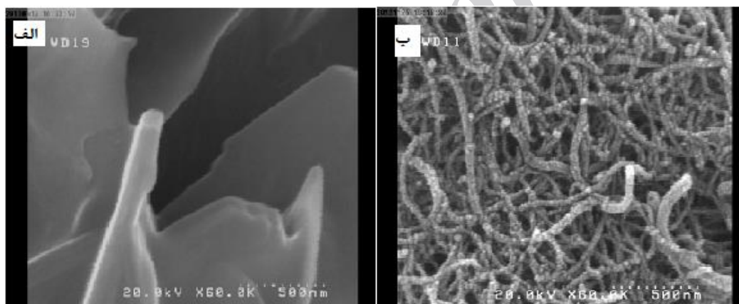
شکل ۱: تصاویر FE-SEM (الف): الکتروُد Ti و (ب): الکتروُد MWCNTs/Ti.
