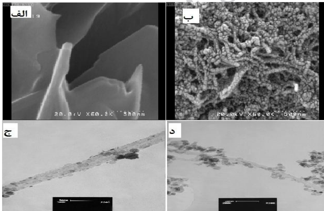
شکل ۶: تصاویر الف): FE-SEM الکتروود تیتانیم (Ti)، ب) FE-SEM الکتروود MWCNTs-TiO 2 /Ti، ج و د) تصاویر TEM الکتروود MWCNTs-TiO 2 /Ti.
