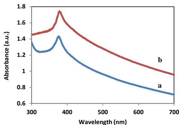
شکل ۶: طیف UV-Vis نانوذرات سنتز شده در دمای (الف) ۴۰۰ و (ب) ۵۰۰ °C.
