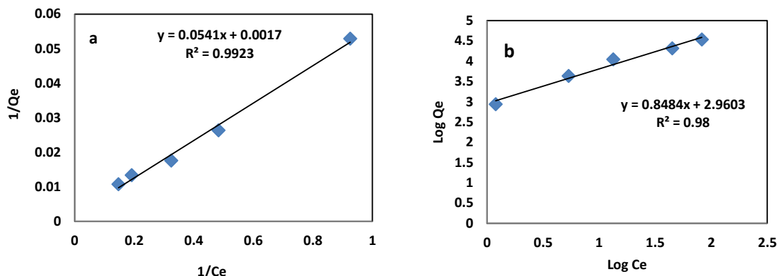
شکل ۹: مدل ایزوترم لانگمویر (a) و فرنلج (b).
