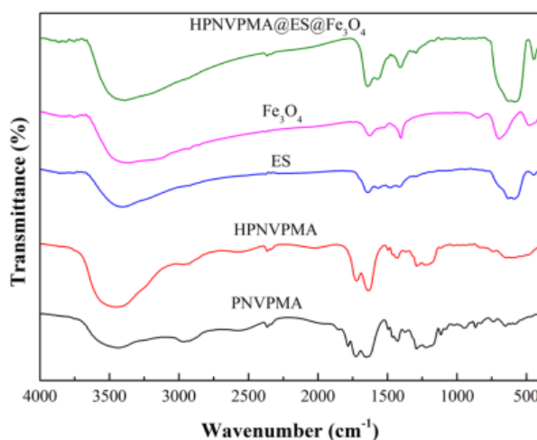
شکل ۲: طیف FT-IR مربوط به HPNVPMA، PNPMA، ES، Fe 3 O 4 و HPNVPMA@ES@Fe 3 O 4
