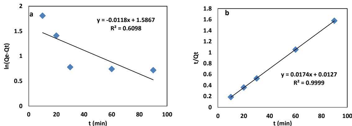
شکل ۱۰: مدل سینتیک (a) مرتبه اول و (b) مرتبه دوم.
