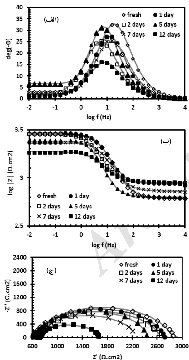
شکل ۳: منحنی‌های (الف) بد-فاز، (ب) بد-مدول و (ج) نایکوئیست نمونه‌های فولادی پس از ۳۰ دقیقه غوطه‌وری در محلول اسیدشویی بدون آب اکسیژنه.
