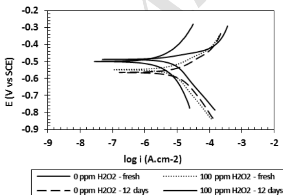
شکل ۷: منحنی پلاریزاسیون نمونه‌های فولادی پس از ۳۰ دقیقه غوطه‌وری در محلول‌های سولفوریک اسید با و بدون آب اکسیژنه.
