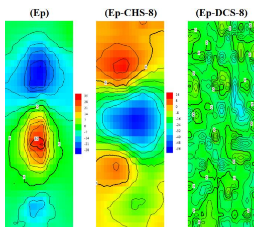
شکل ۴: تصاویر نقشه‌های جریان‌های کاتدی و آندی در ناحیه اطراف خراش برای پوشش‌های مختلف بعد از ۲۴ ساعت غوطه‌وری در محلول ۰.۳٪ وزنی از NaCl. واحد چگالی جریان \mu\text{A}\cdot\text{cm}^{-2} و مساحت سطح رویش شده 1 \times 2 \text{ mm}^2 .
