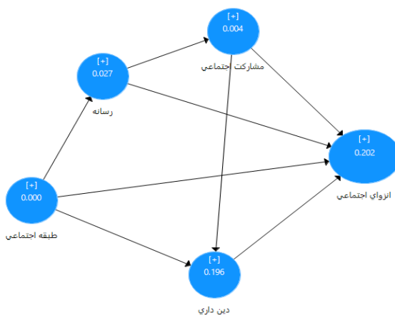
نمودار ۳. مقادیر معیار استون-گیسر برای متغیرهای درون‌زا (Q2)
