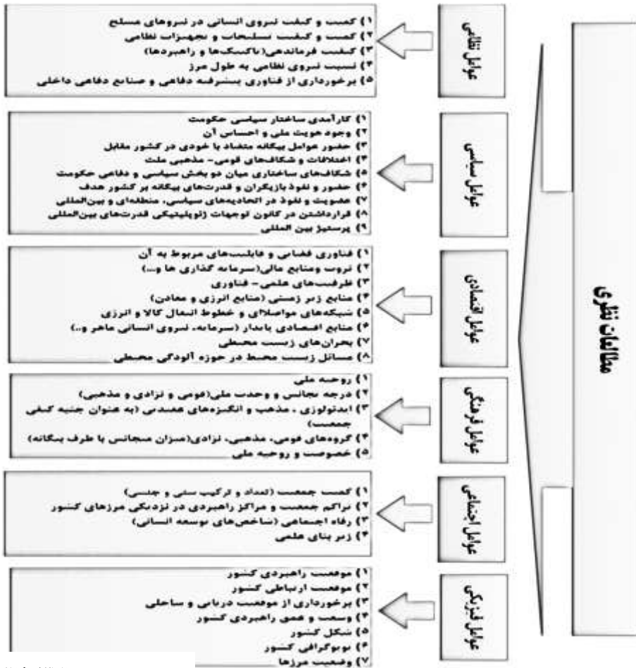
شکل ۲: عوامل کلان ژئوپلیتیکی
