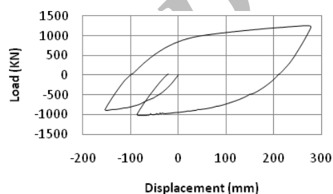
الف) رفتار هیستریسیس قاب خالی - Bare Frame
