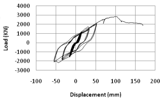
ج) رفتار هیستریسیس قاب دارای میانقاب مشابه EIF-2
