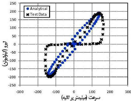
نمودار (۴): نمودار نیرو-جابجایی و نمودار نیرو-سرعت، آزمایش ۱ هرتز
