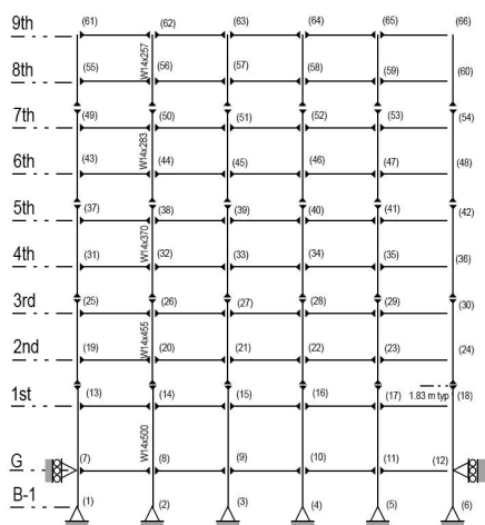
شکل (۹): پلان و قاب خمشی شمالی - جنوبی
