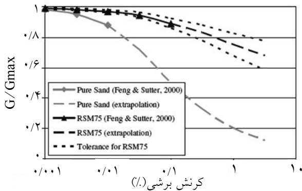
شکل (۴): منحنی کاهش مدول برشی [۷]
