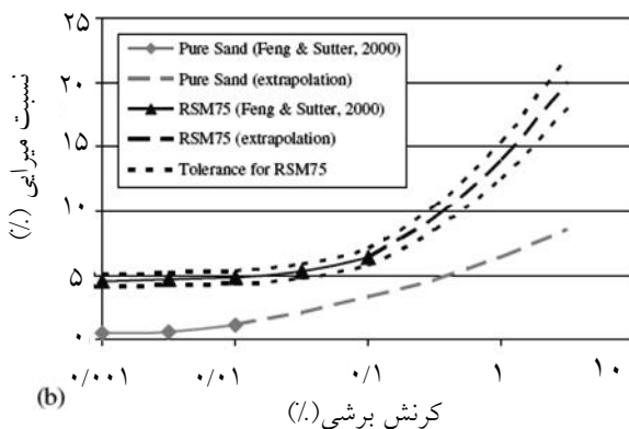
شکل (۵): منحنی نسبت میرایی [۷]
