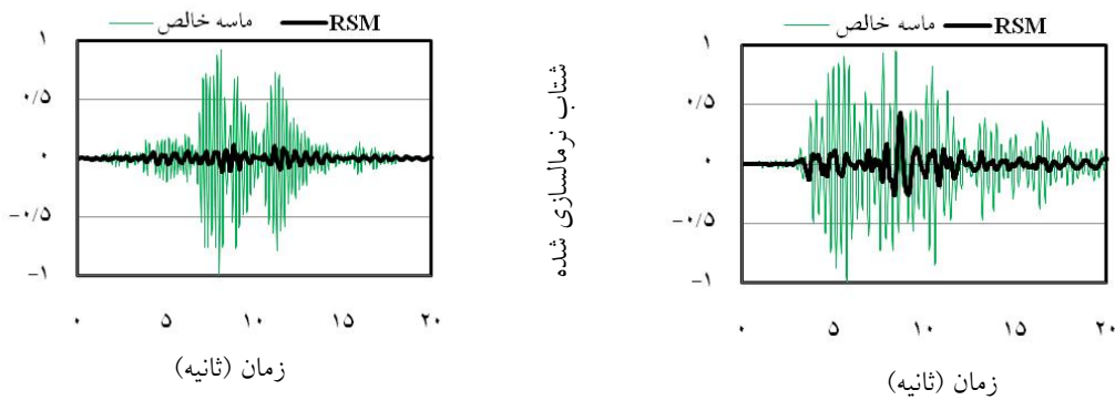
شکل (۷): نتایج شبیه‌سازی مجدد مدل مرجع تیسانگ
