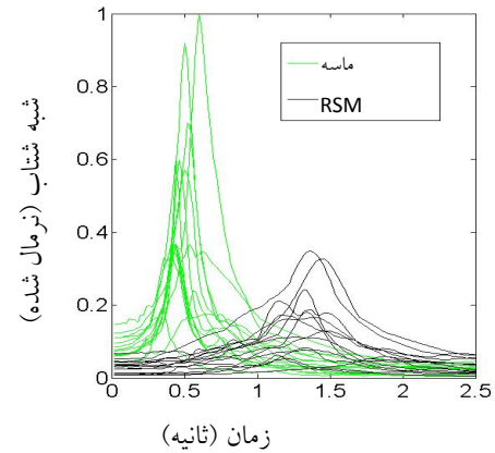
شکل (۱۲): طیف پاسخ شتاب (نرمال شده) زلزله‌های مربوط
