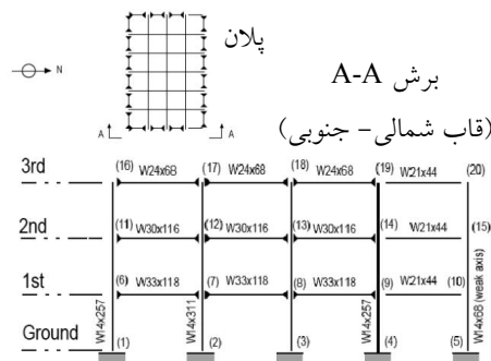
شکل (۸): پلان و قاب خمشی شمالی - جنوبی
