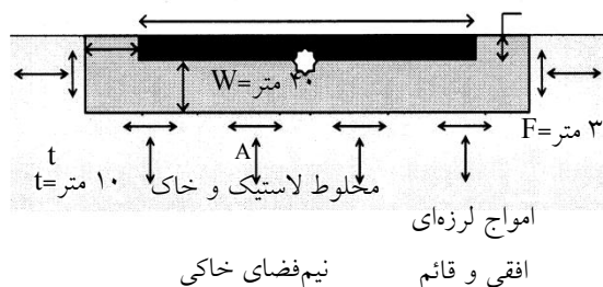
شکل (۲): مدل مرجع در مدلسازی المان محدود [۷]
