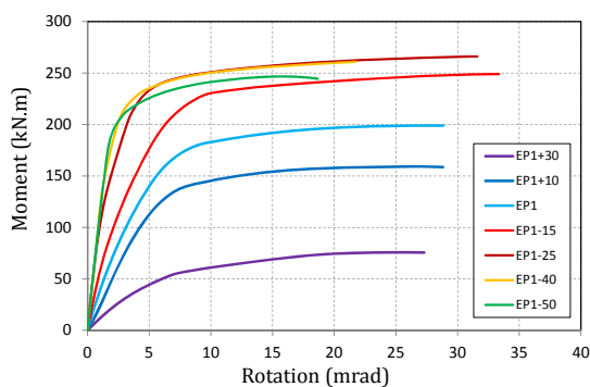
شکل (۲۰): نمودار لنگر خمشی-دوران در اتصال EP1 با نیروی محوری
