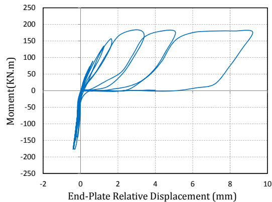
شکل (۲۷): نمودار لنگر خمشی اتصال بر حسب جداسازی صفحه‌ای انتهایی
