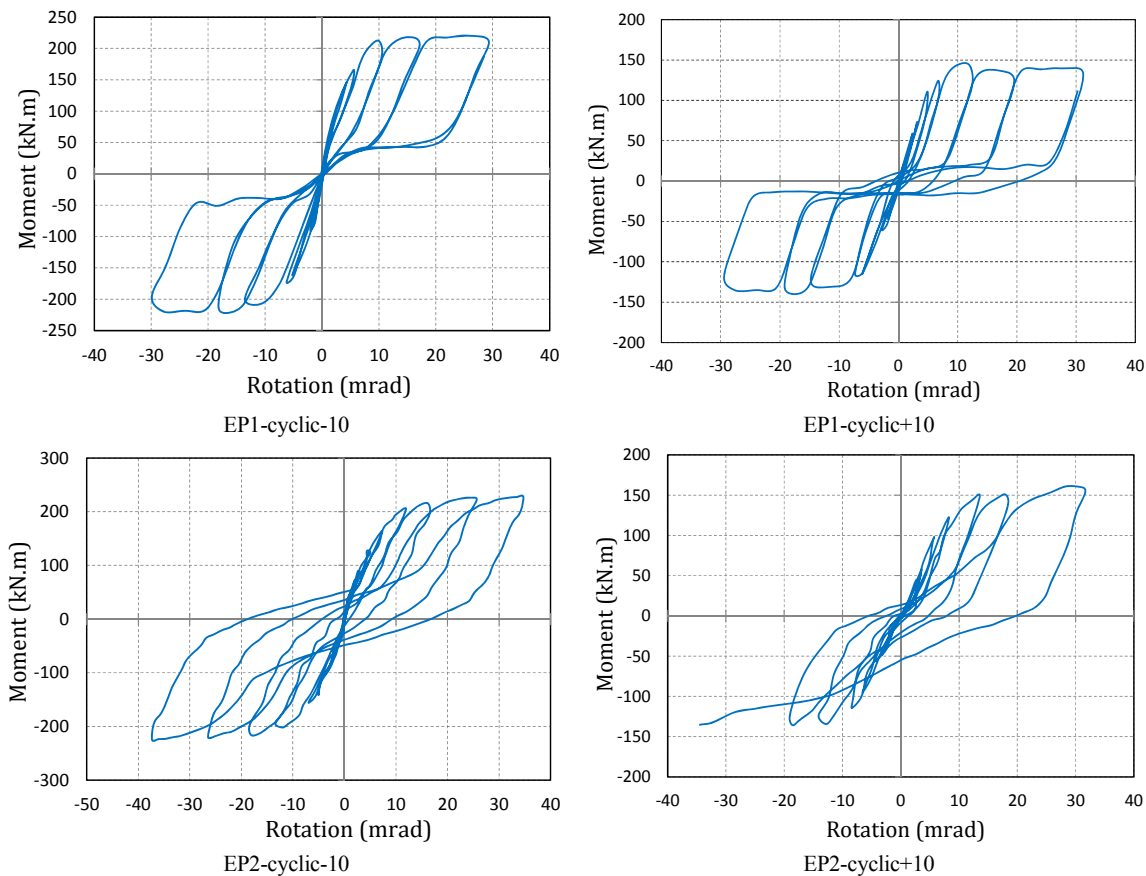
شکل (۳۳): نمودار هیستریزیس اتصال EP1 و EP2
