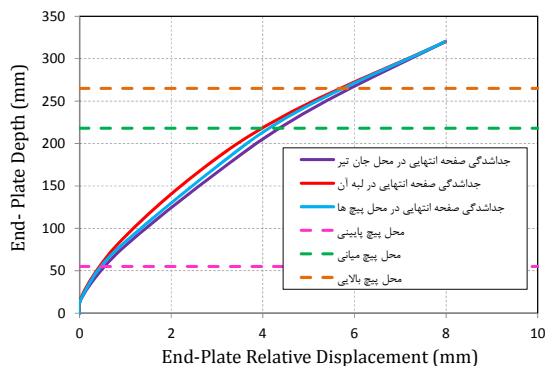
شکل (۹): جداسدگی صفحه‌ی انتهایی اتصال EP1
