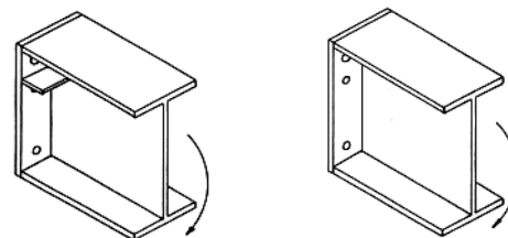
ب) چهارپیچی با سخت‌کننده
