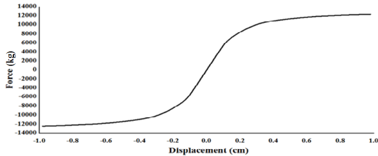
شکل (۴): منحنی نیرو-تغییر مکان المان پیشنهادی
