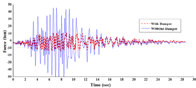
ب) قاب شش طبقه
