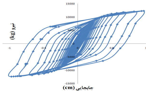
شکل (۵): منحنی هیستریسیس المان پیشنهادی
