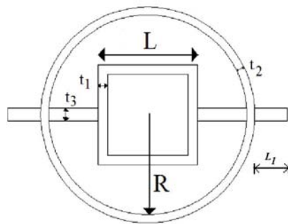
شکل (۱): المان پیشنهادی
