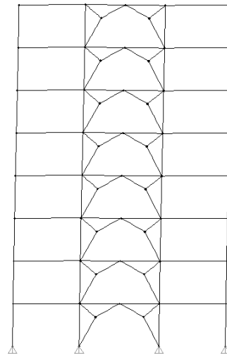
الف) قاب با المان پیشنهادی
