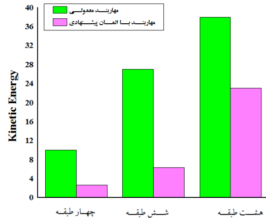
شکل (۱۱): مقایسه انرژی جنبشی در زلزله نورتریج
