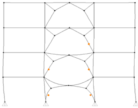
ب) قاب با مهاربند معمولی
