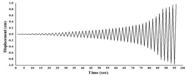
شکل (۳): تاریخچه بارگذاری
