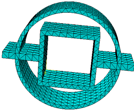
شکل (۲): نمایش مش بندی المان پیشنهادی
