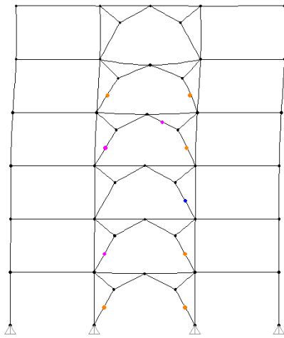
ب) قاب با مهاربند معمولی
