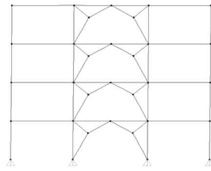
الف) قاب با المان پیشنهادی
