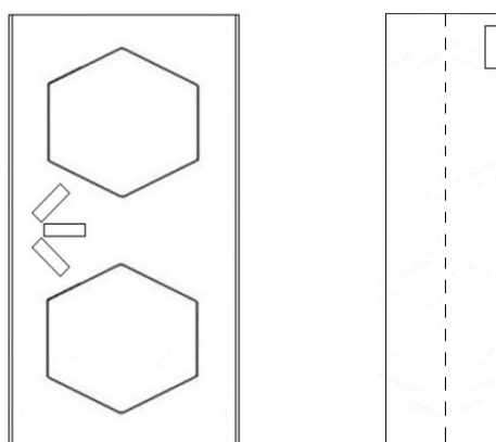
شکل (۹): نمایش محل کرنش سنج‌های نصب شده بر روی بال و جان
