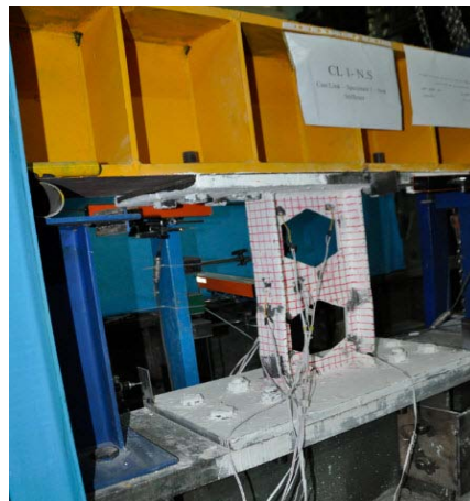
شکل (۱۴): نمایش گسیختگی نمونه شماره یک
