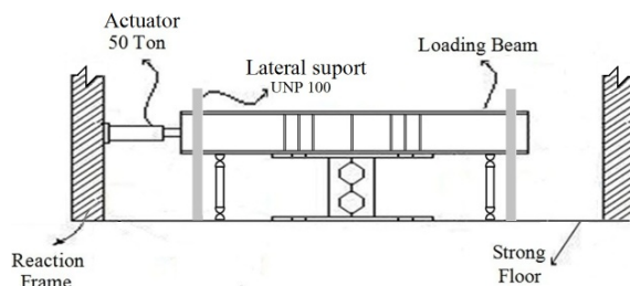
شکل (۶): پیکربندی نمونه‌ها جهت آزمایش
