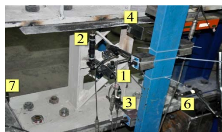
شکل (۹): نمایش محل کرنش سنج‌های نصب شده بر روی بال و جان
