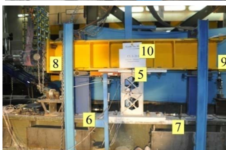
شکل (۱۰): نمایش برخی از تغییر مکان سنج‌های نصب شده بر روی نمونه‌های آزمایشگاهی
