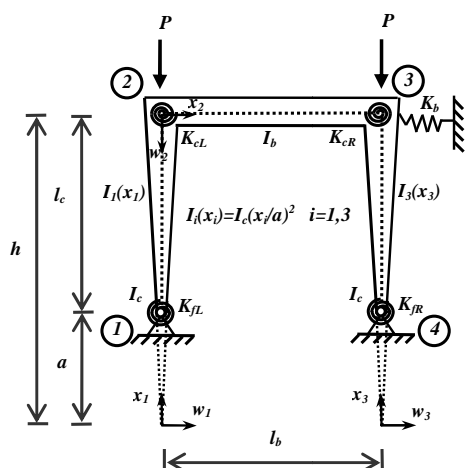
ب- قاب ساده‌ی نامنشوری
