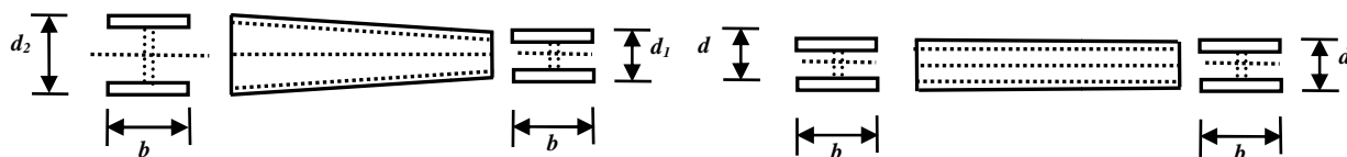
ب- پهنا‌ی بال ثابت و بلندای جان متغیر (نامنشوری)
