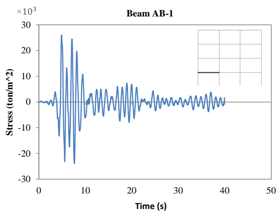
شکل (۵): تاریخچه زمانی تنش تیر AB-1 تحت زلزله لوماپریتا
