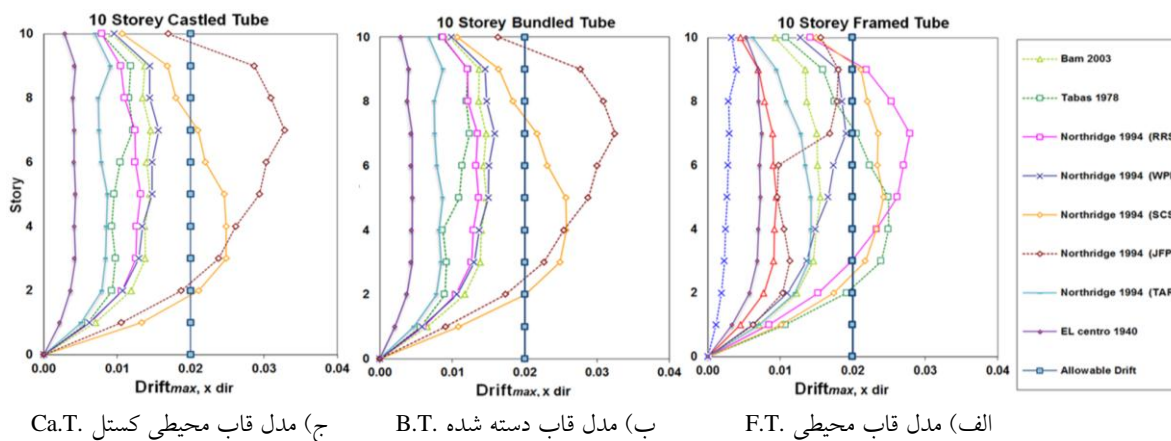
شکل (۱۰): پوش ماکزیمم دریفت طبقات
