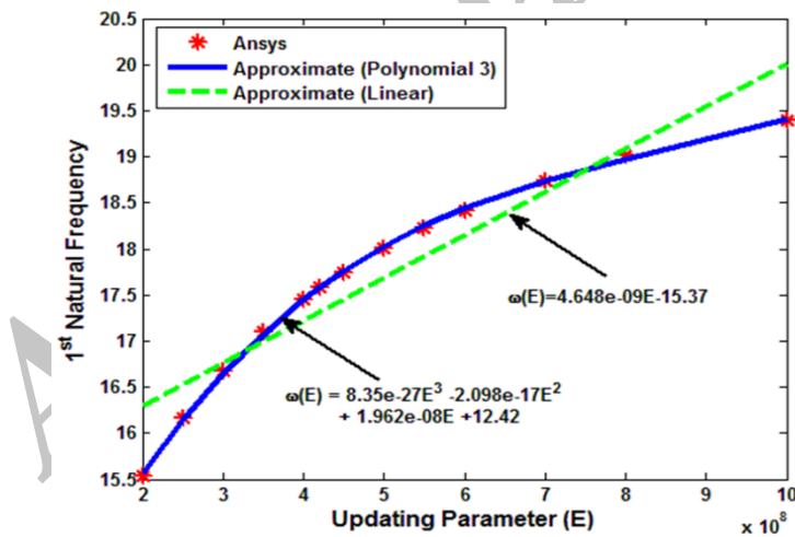
شکل ۶- نمودار برازش درجه سه و خطی فرکانس طبیعی اول
