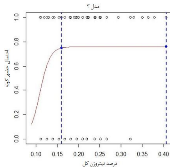
شکل ۱۱: برازش تابع HOF به متغیر نیتروژن کل
