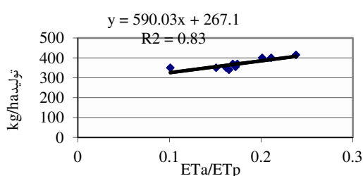
شکل ۳- ارتباط بین تولید سالانه علوفه و تبخیر و تعرق واقعی به تبخیر و تعرق پتانسیل در مرتع حوزه شیرکوه
