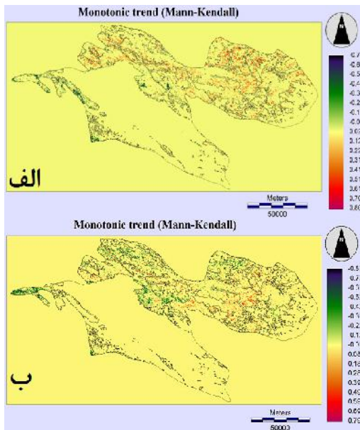
شکل ۷: نقشه مناطق دارای روند معنی‌دار شروع فصل رشد (الف) و پایان فصل رشد (ب) (p=0.05) برای ۱۵ فصل
