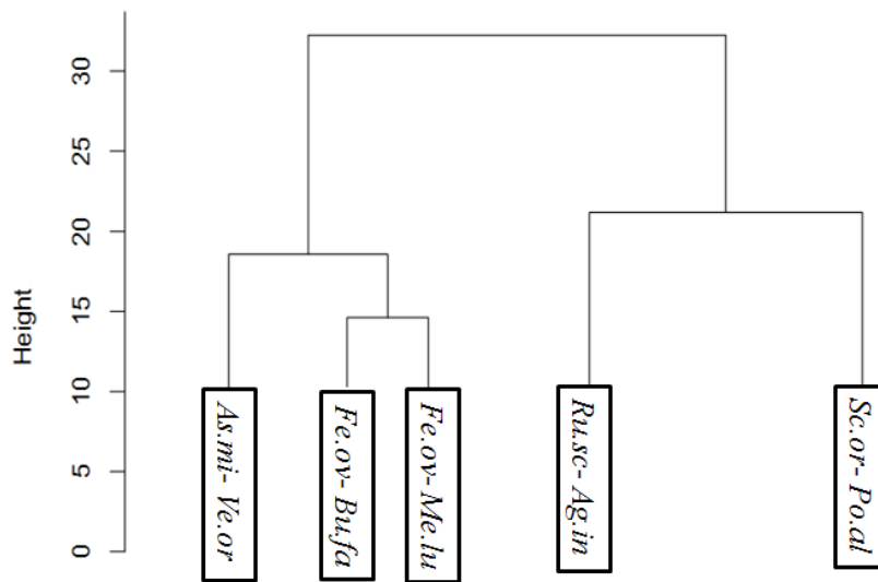
شکل ۲: دیاگرام طبقه‌بندی پوشش گیاهی در محدوده معدن مس سونگون (هر زیراجتماع بر اساس دو گونه غالب مشخص شده است) (Me.lu) ، Bupleurum falcatum ( Bu.fa )، Festuca ovina ( Fe.ov )، Verbascum oreophilum ( Ve.or )، Astragalus microcephalus ( As.mi ) (Po.al) ، Scariola orientalis ( Sc.or )، Agropyron intermedium ( Ag.in )، Rumex scutatus ( Ru.sc )، Medicago lupulina
