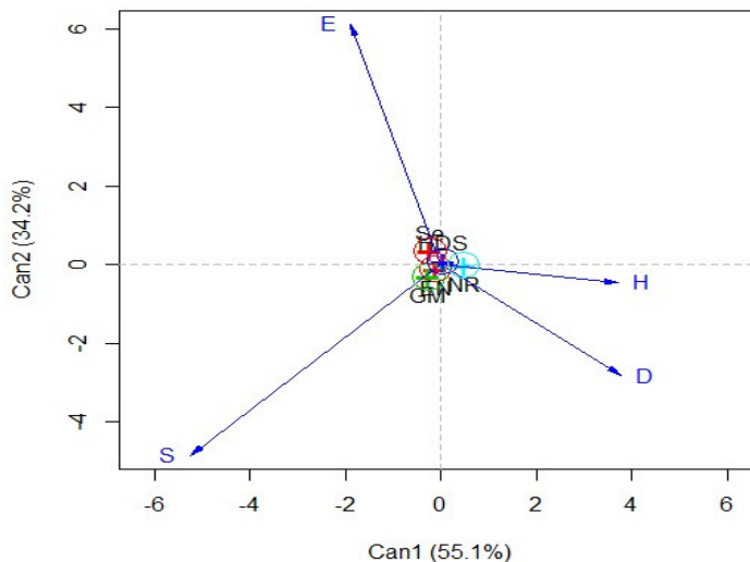
شکل ۲: نتایج حاصل از آنالیز تشخیص کانونیک تعمیمی (GCCA) در تیمارهای مختلف بیولوژیک بر روی شاخص‌های تنوع گونه‌ای: GM مدیریت چرا، NR: مرتع طبیعی، S: بذرپاشی، HDS: کپه کاری، EX: فرق، S غنای گونه‌ای، H: شاخص شانون واینر، E: شاخص یکنواختی، D: شاخص سیسمپسون هستند.
