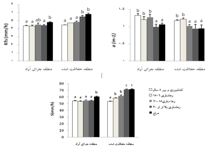
شکل ۱: تاثیر رهاسازی مختلف در مدیریت چرای حیوانات بر ضریب هدایت هیدرولیکی خاک (kfs)، عکس طول درشت موینگی (a) و ضریب جذب خاک (s)
