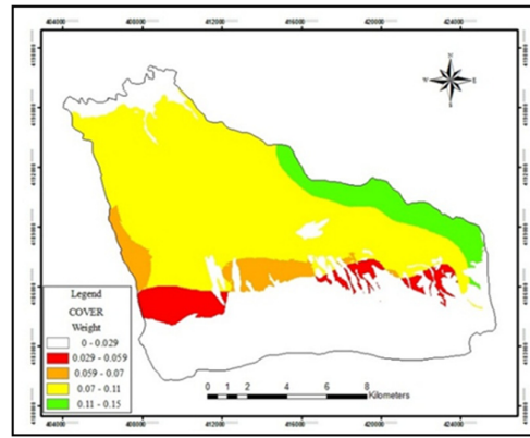
شکل ۱۰: نقشه اهمیت نسبی مکانی در معیار پوشش گیاهی
