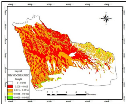
شکل ۹: نقشه اهمیت نسبی مکانی در معیار فیزیوگرافی
