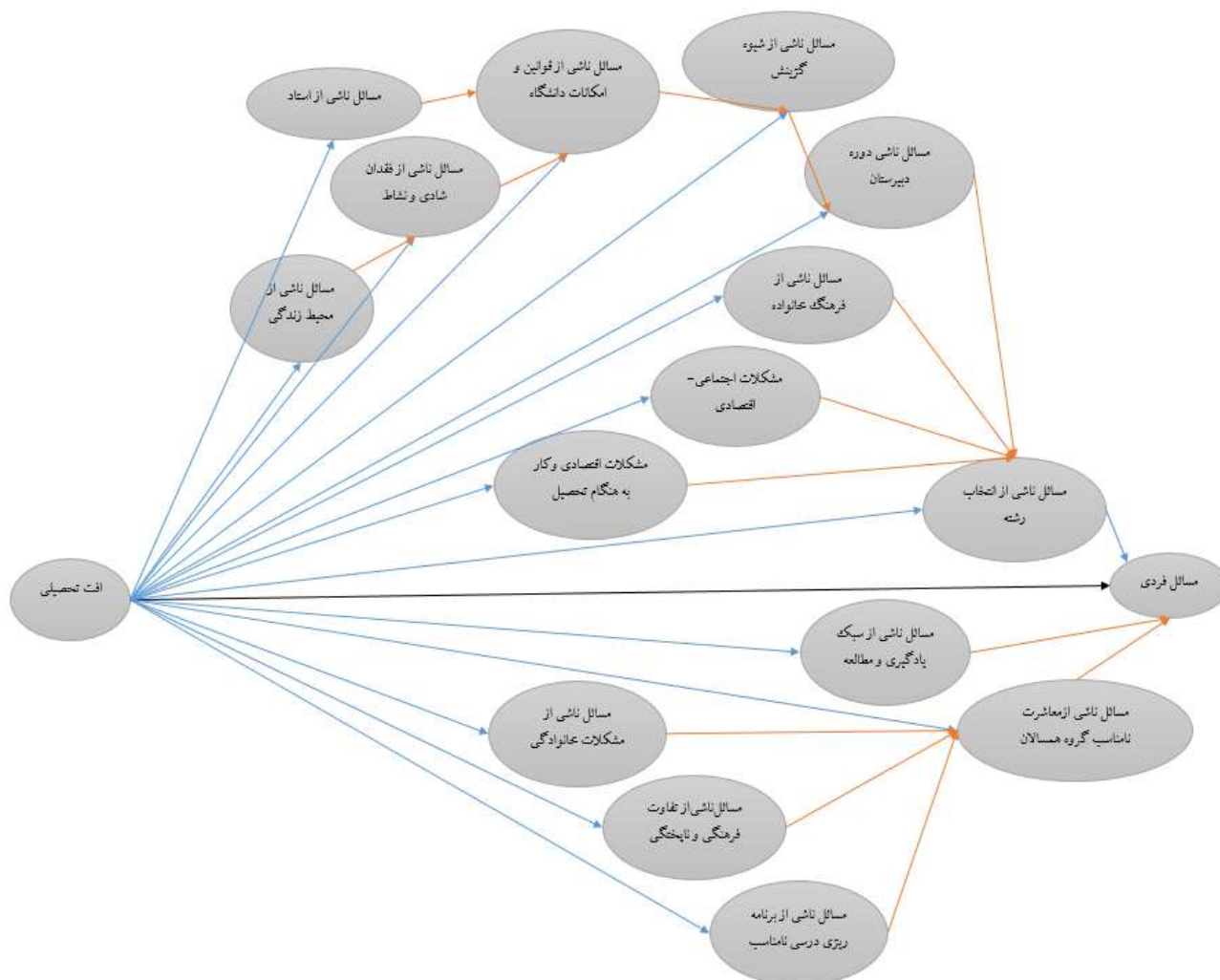
شکل ۱. مدل شبکه بیزی داده‌ها
