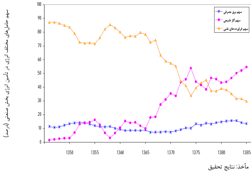
نمودار 2: نمودار سهم مصرف برق، گاز طبیعی و فرآورده‌های نفتی از کل مصرف انرژی بخش صنعتی
