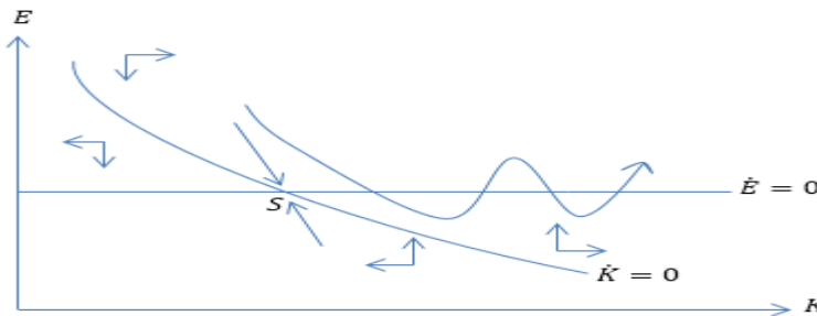
شکل ۳: انتقال های پویا و تعادل های چندگانه Fig.3. Transitional dynamics and multiple equilibrium
