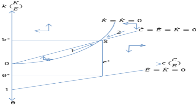
شکل ۱: ارزش های بهینه و وضعیت پایدار Fig.1. Steady state and optimal values
